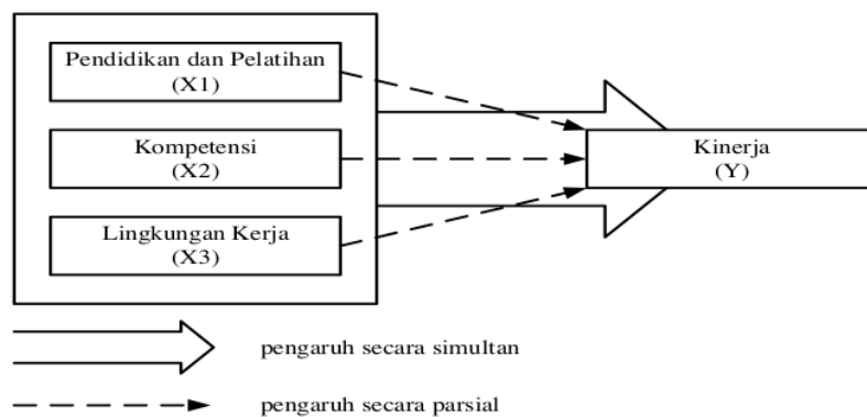
Gambar 1. Kerangka Pemikiran
