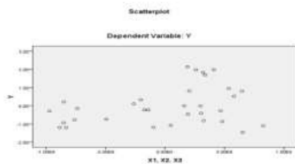
Gambar 2. Uji Heteroskedastisitas
