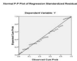
Gambar 1. Uji Normalitas Distribusi
