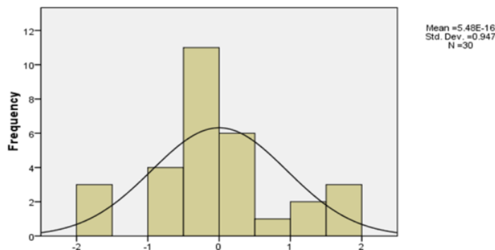
Gambar 1. Grafik Histogram
