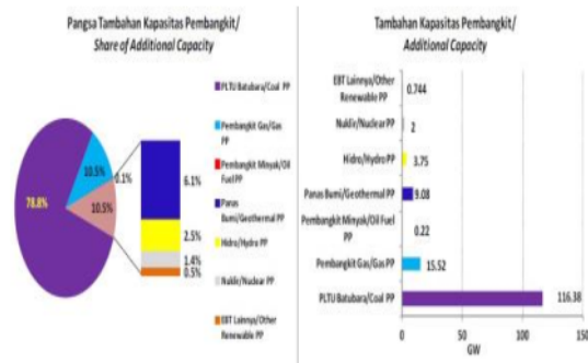
Gambar 3 Rencana tambahan kapasitas pembangkit listrik Indonesia dalam rentang waktu 2010-2030
