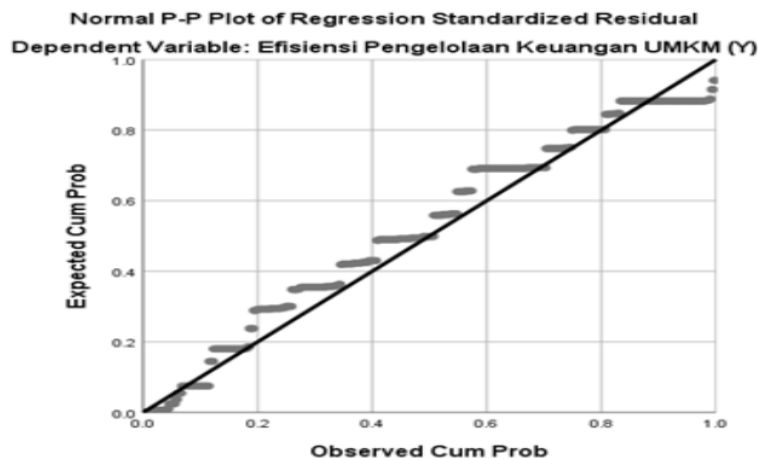
Gambar 1. Analisis normalitas
