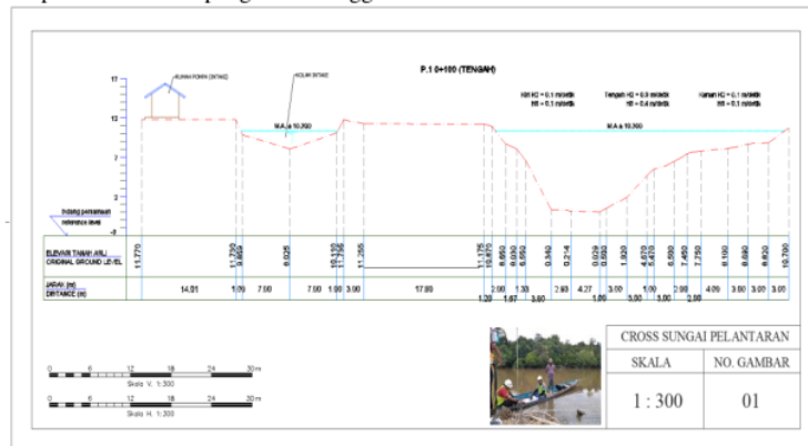
GAMBAR 4 PENGUKURAN DEBIT SESAAT PADA INTAKE CEMPAGA
