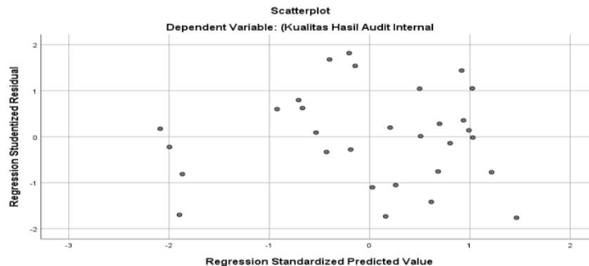
Gambar 2. Uji Asumsi Heteroskedastisitas
