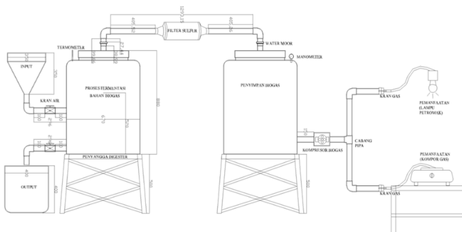
Gambar 2. Rancangan Digester Limbah Cair Tahu (12)
