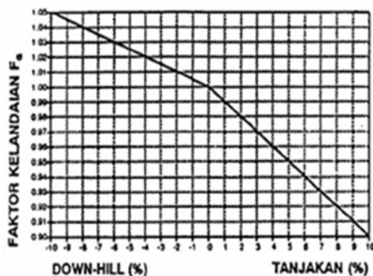
Gambar 1. Grafik faktor penyesuaian untuk kelandaian Sumber: MKJI, 1997
