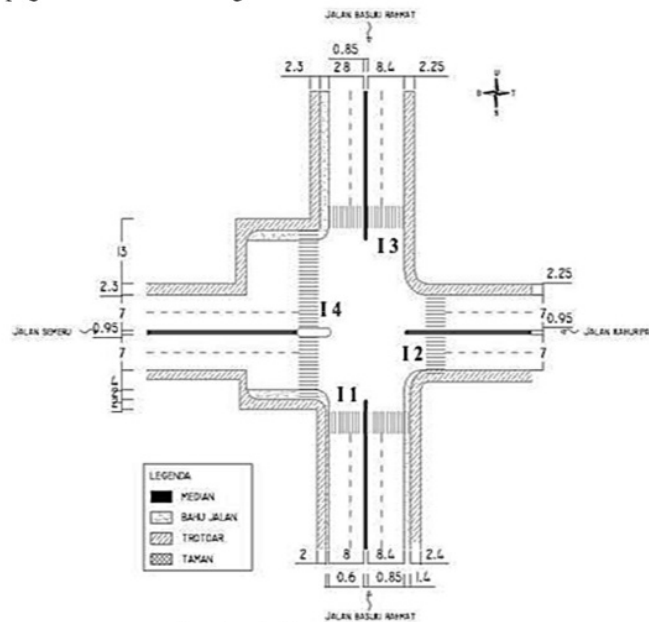
Gambar 8. Geometrik Perimpangan Sumber: Hasil Analisa, 2020
