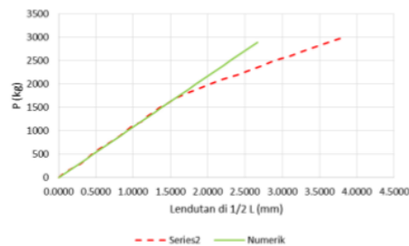
Gambar 12. Perbandingan P vs Δ Hasil Eksperimen, Analitis dan Numerik pada balok BK
