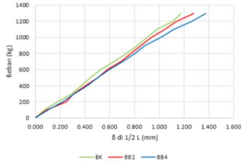
Gambar 6. Grafik Hubungan Beban dan Lentutan pada Kondisi Praretak
