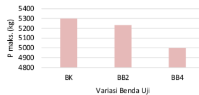
Gambar 7. Perbandingan Beban Ultimit Masing-Masing Variasi
