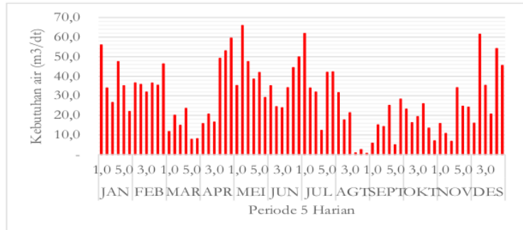
Gambar 8. Kebutuhan Air PTT Rencana (300%).
