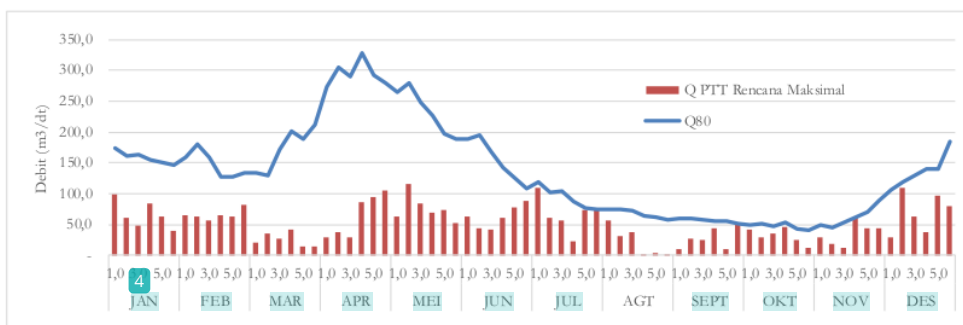
Gambar 10. Neraca Air PTT Rencana Maksimal
