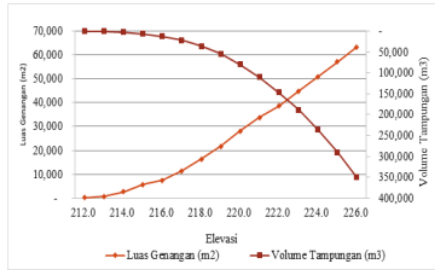
Gambar 11. Lengkung Kapasitas
