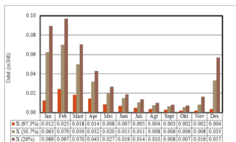
Gambar 12. Debit Adalan Berbagai kondisi
