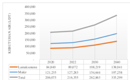
Gambar 8. Kebutuhan Air Penduduk
