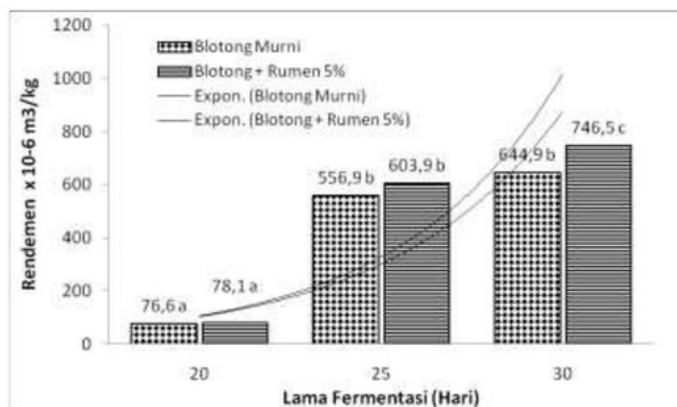
Gambar 2. Grafik rendemen biogas yang dihasilkan dari blotong limbah PG. Krebet dalam \text{m}^3/\text{kg} . Notasi berbeda menunjukkan beda nyata pada \alpha=5\%
