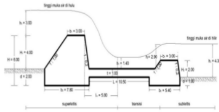
Gambar 4. Sketsa dimensi check dam
