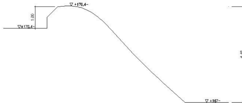
Gambar 2. Dimensi Bendung
