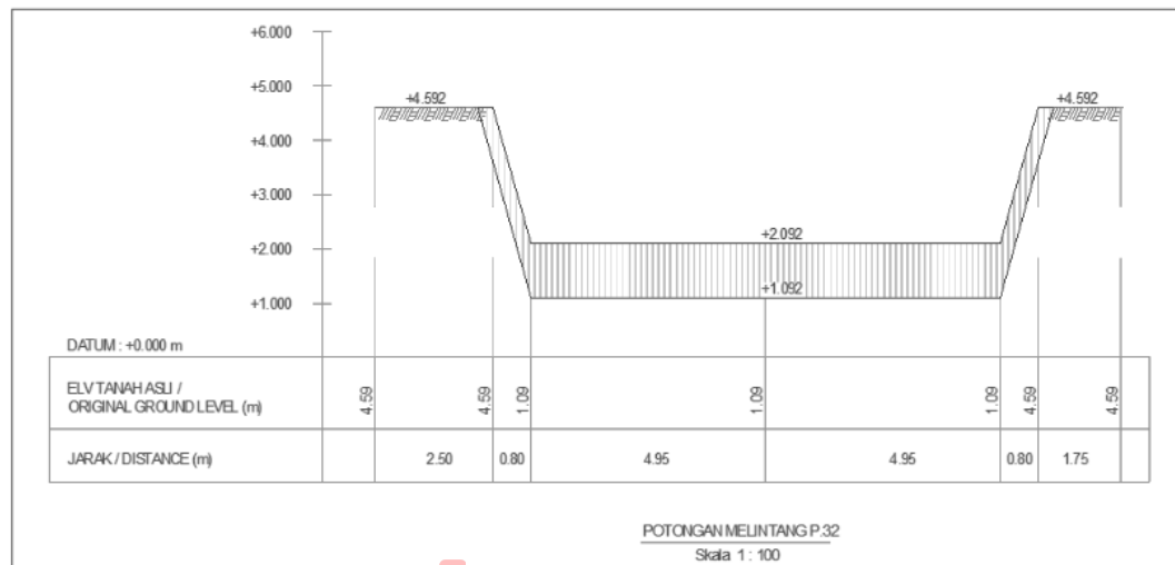
Gambar 3 Bentuk tipikal saluran
