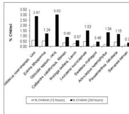
Gambar 2. Kadar CH 4 (%) per ml produksi gas pada waktu pengamatan 12 dan 24 jam dari 10 jenis daun tanaman secara in-vitro .
